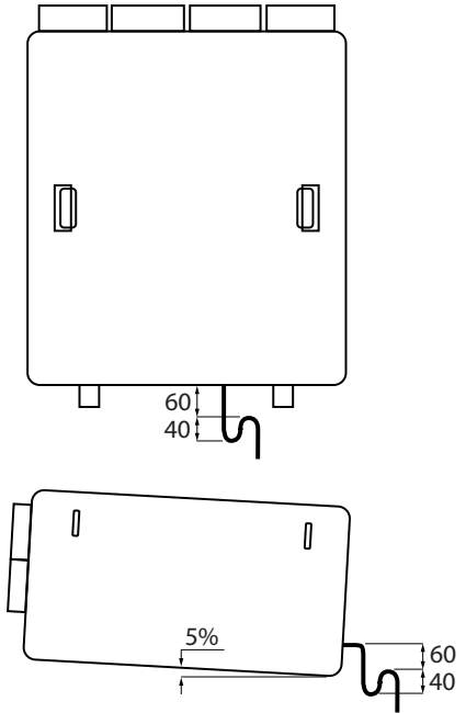
Рис. 5 Сифон на скроплины в КСХ и похлыение версии подвешиваемой.
