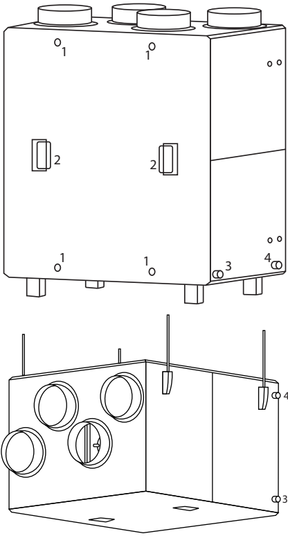
Рис. 3 Установка для обработки воздуха КСХ в стоячем и подвешенном рабочем положениях. Для снятия передней панели необходимо снять четыре зажима (1). Одновременно необходимо придержать рукоятки панели (2). См. обозначения на рис. 3.
