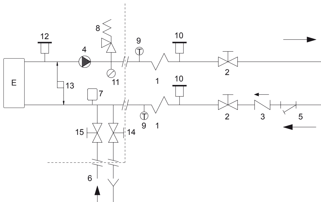
Schemat podłączania obiegu wodnego Hydraulic circuit connection diagram
