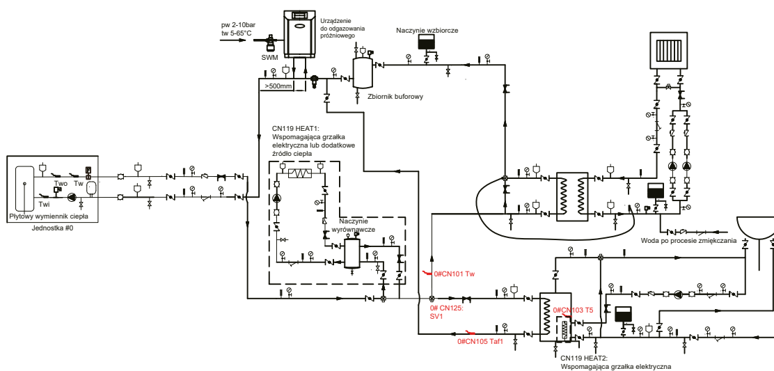
Schemat nr 2. Pojedyncze urządzenie z wymiennikiem płytowym
